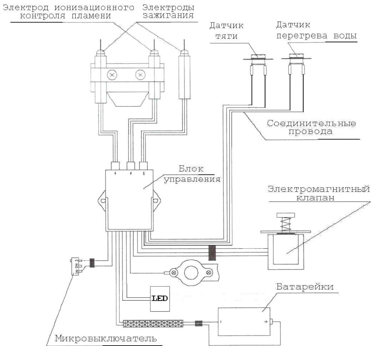
Рис. 2.Схемаэлектрическая
